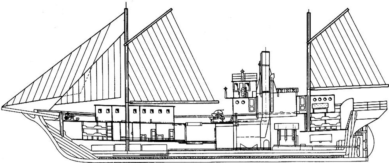
Научно-исследовательское судно «Персей» (рисунок) и схематический разрез внутреннего обустройства
